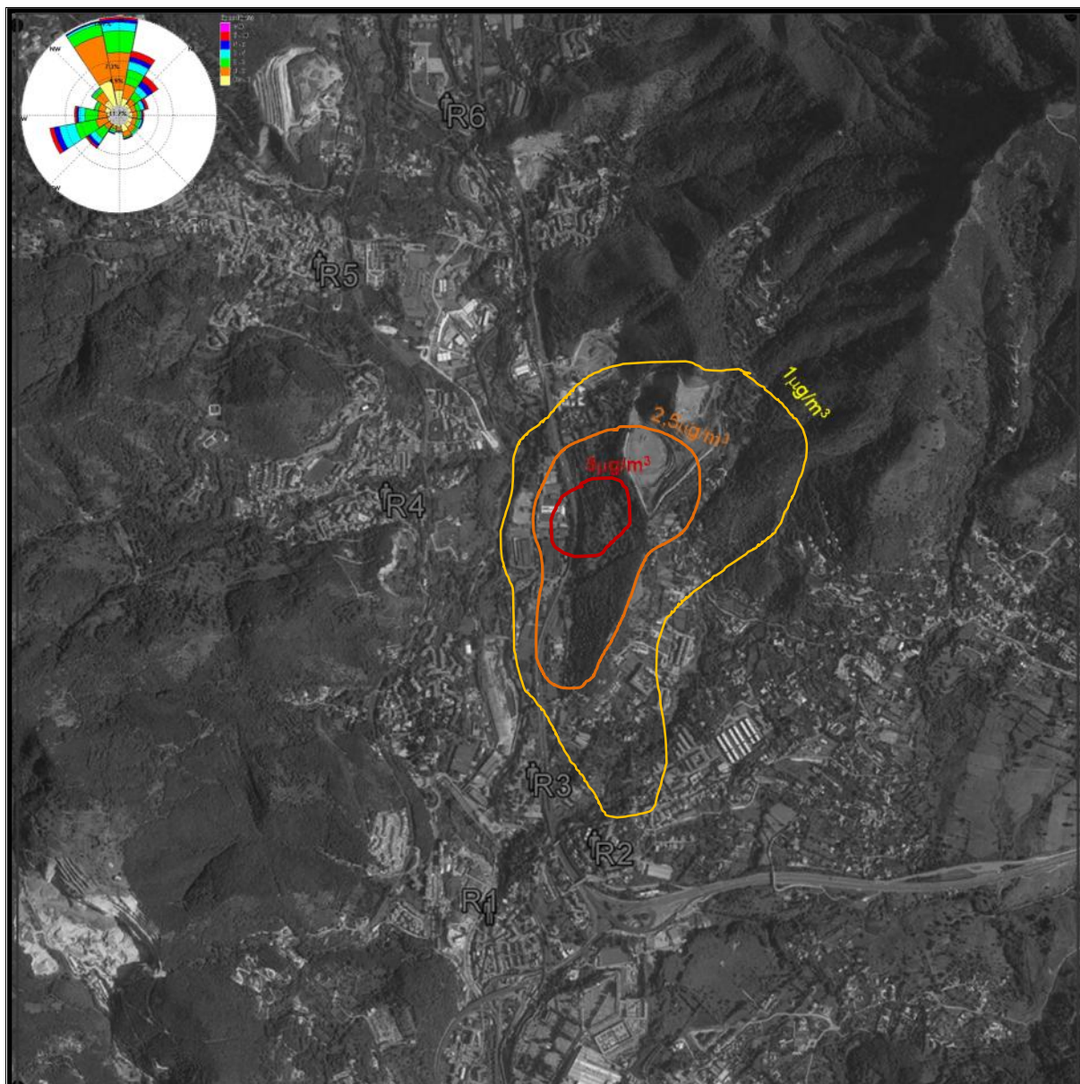
Figura 4.16 – mappa della concentrazione media annua al suolo di PTS in riferimento allo scenario massivo emissivo delle Fonderie Pisano.
