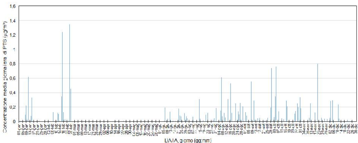
Figura 4.4 –andamento nel tempo della concentrazione media giornaliera di PTS, espressa in \mu\text{g}/\text{m}^3 , al bersaglio R4, nello scenario di esercizio ordinario.
