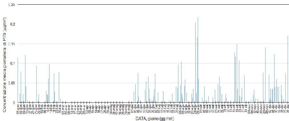
Figura 4.1 –andamento nel tempo della concentrazione media giornaliera di PTS, espressa in \mu\text{g}/\text{m}^3 , al bersaglio R1, nello scenario di esercizio ordinario.
