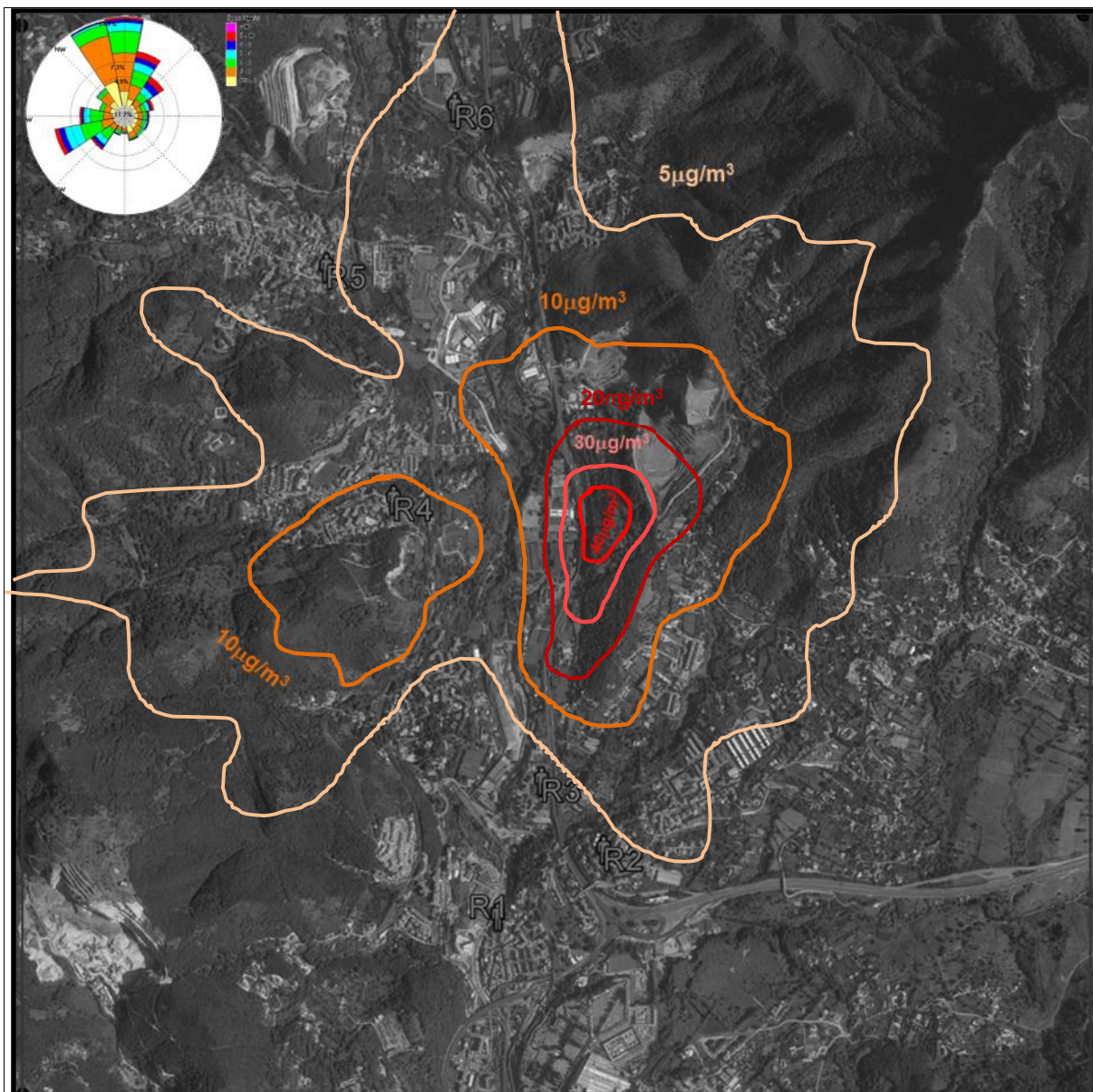
Figura 4.15 – mappa della massima concentrazione giornaliera al suolo di PTS in riferimento allo scenario massimamente emissivo delle Fonderie Pisano.
