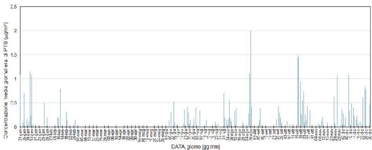
Figura 4.7 –andamento nel tempo della concentrazione media giornaliera di PTS, espressa in \mu\text{g}/\text{m}^3 , al bersaglio R1, nello scenario massimo emissivo.
